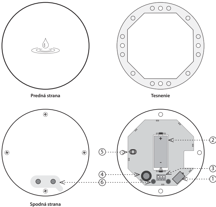
Spodná strana
